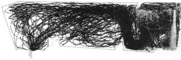
图 3 中间包内夹杂物运动迹线图 Fig. 3 Moving trace of inclusions in tundish
